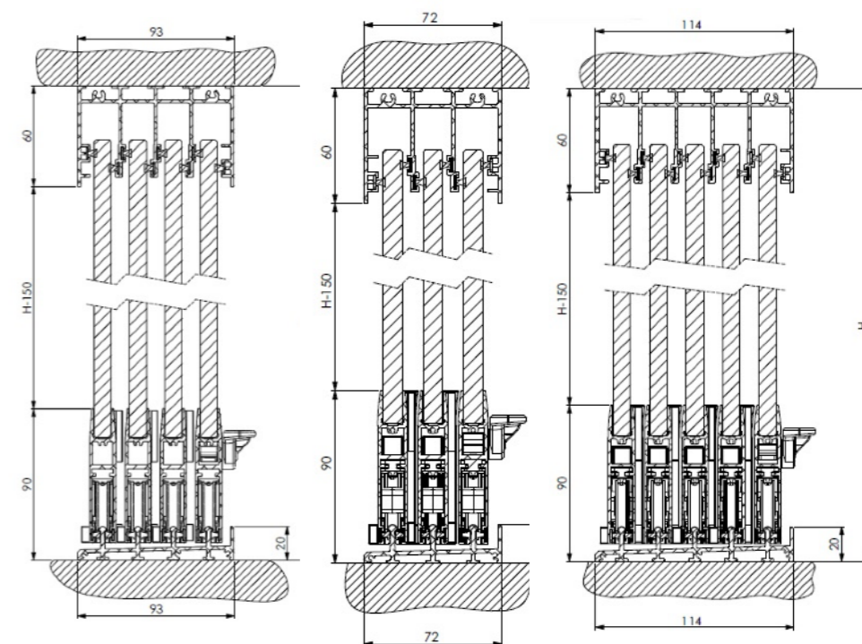
▲ ukázka šířky systémů při 3 či 4 nebo 5 kolejkách
