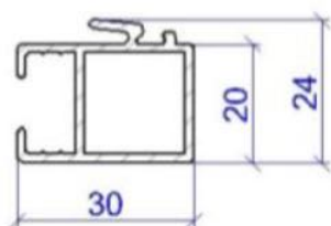
Profil vertikální Plus
