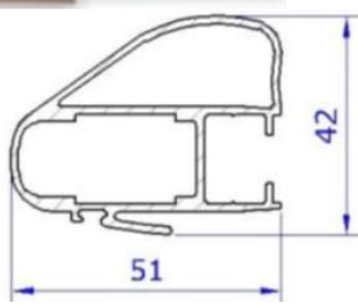
Zesílený profil "s boulí"
