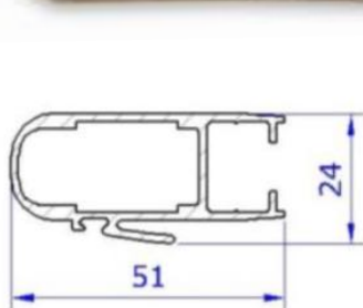
Profil vertikální Combi
